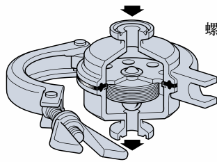
卡箍式连接
