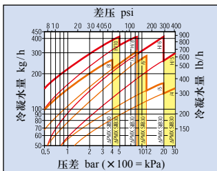
SIB30排量
