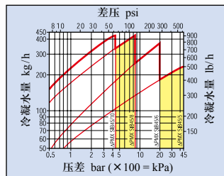
SIB45排量
