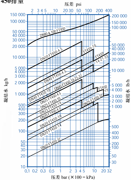
FT450排量
