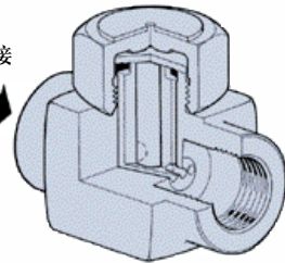
BTD52L
