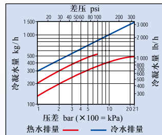
TSS21排量
