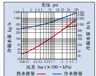
SBP30排量
