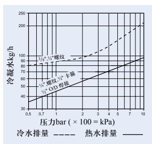
BTD52L排量
