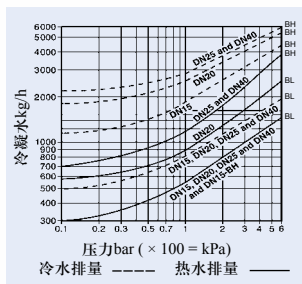
BT6-B排量
