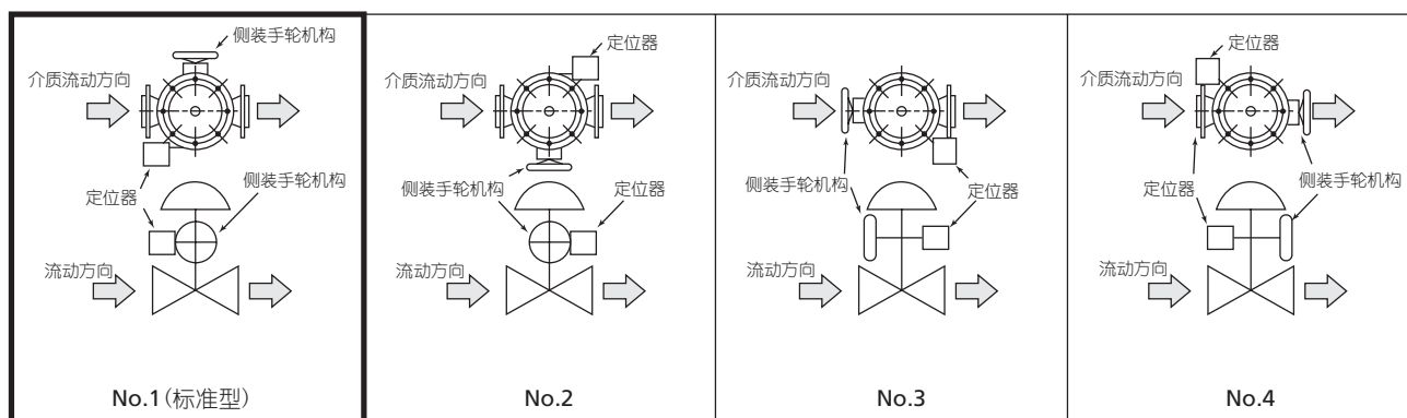
图 7 配管安装示意图
