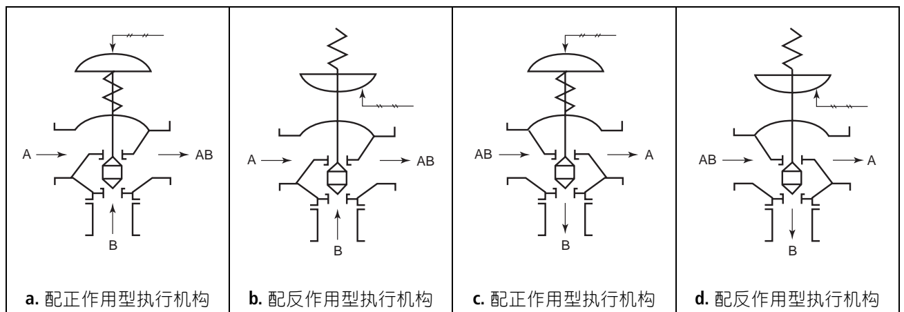
图 3 阀作用
