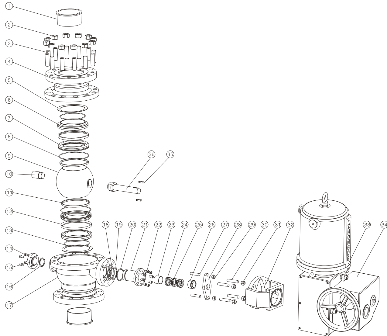
图2 耐磨球阀主要零部件分解图
