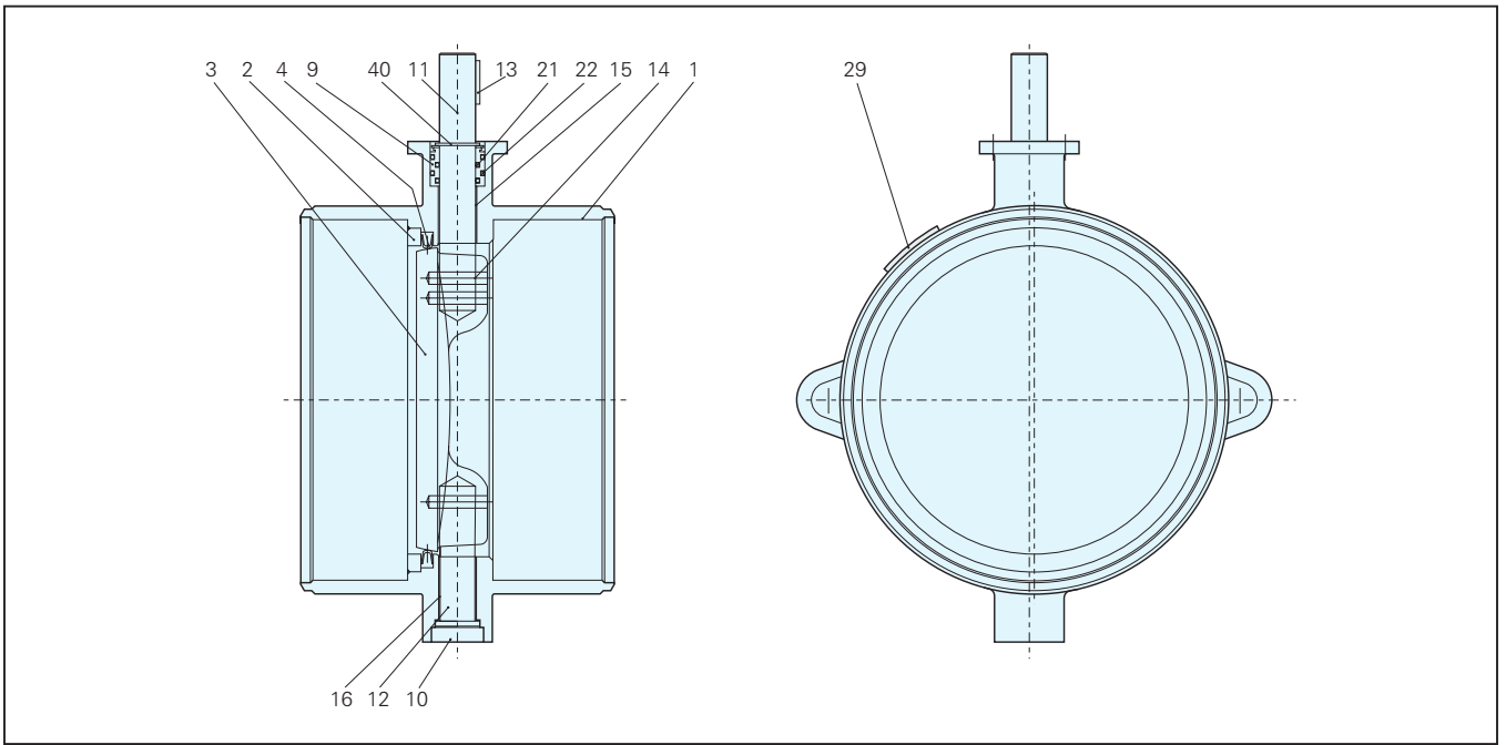
标准型L90阀门零部件名称及材料
