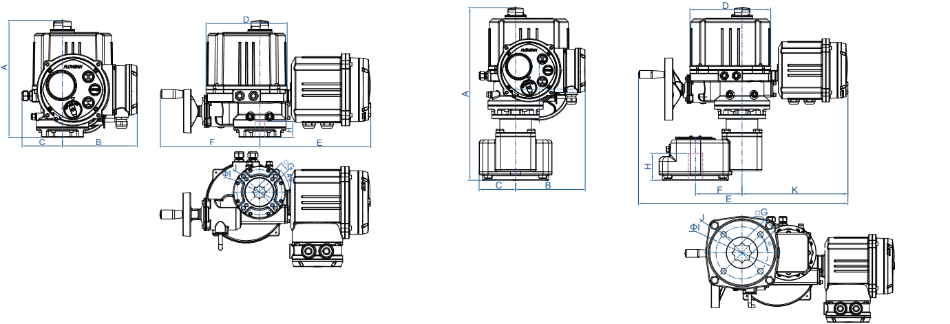
EOH10-150EOH200-500
