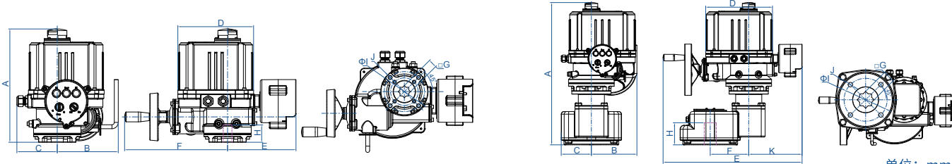
S4(EOH10-150)S4(EOH200-500)
