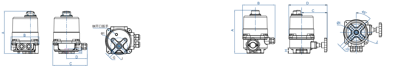
EOH10-150EOH200-500
